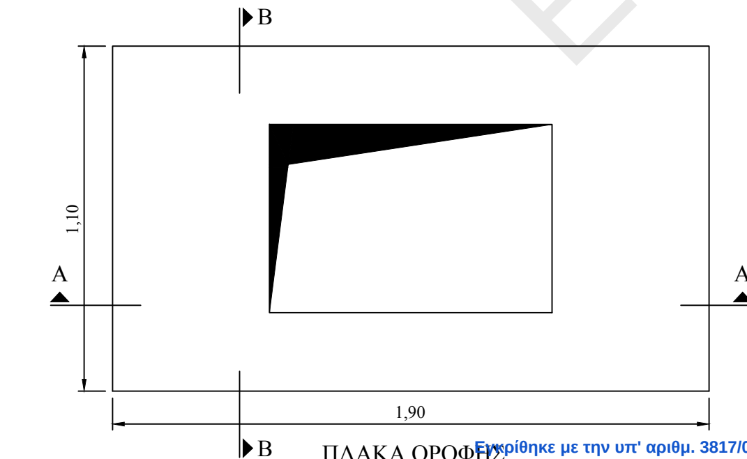
ΚΑΤΟΨΗ
