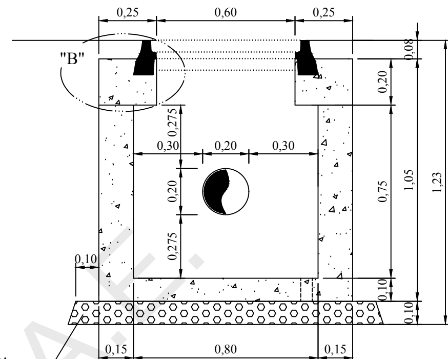
ΤΟΜΗ Β-Β
