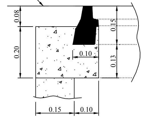
ΛΕΠΤΟΜΕΡΕΙΑ "Β"
