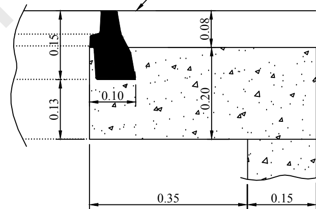
ΛΕΠΤΟΜΕΡΕΙΑ "Α"
