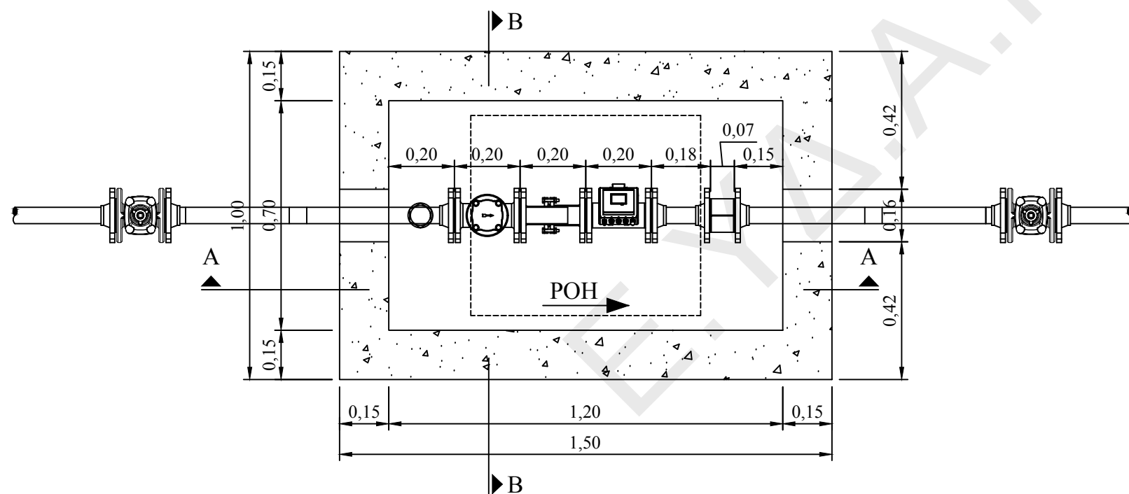
ΚΑΤΟΨΗ
