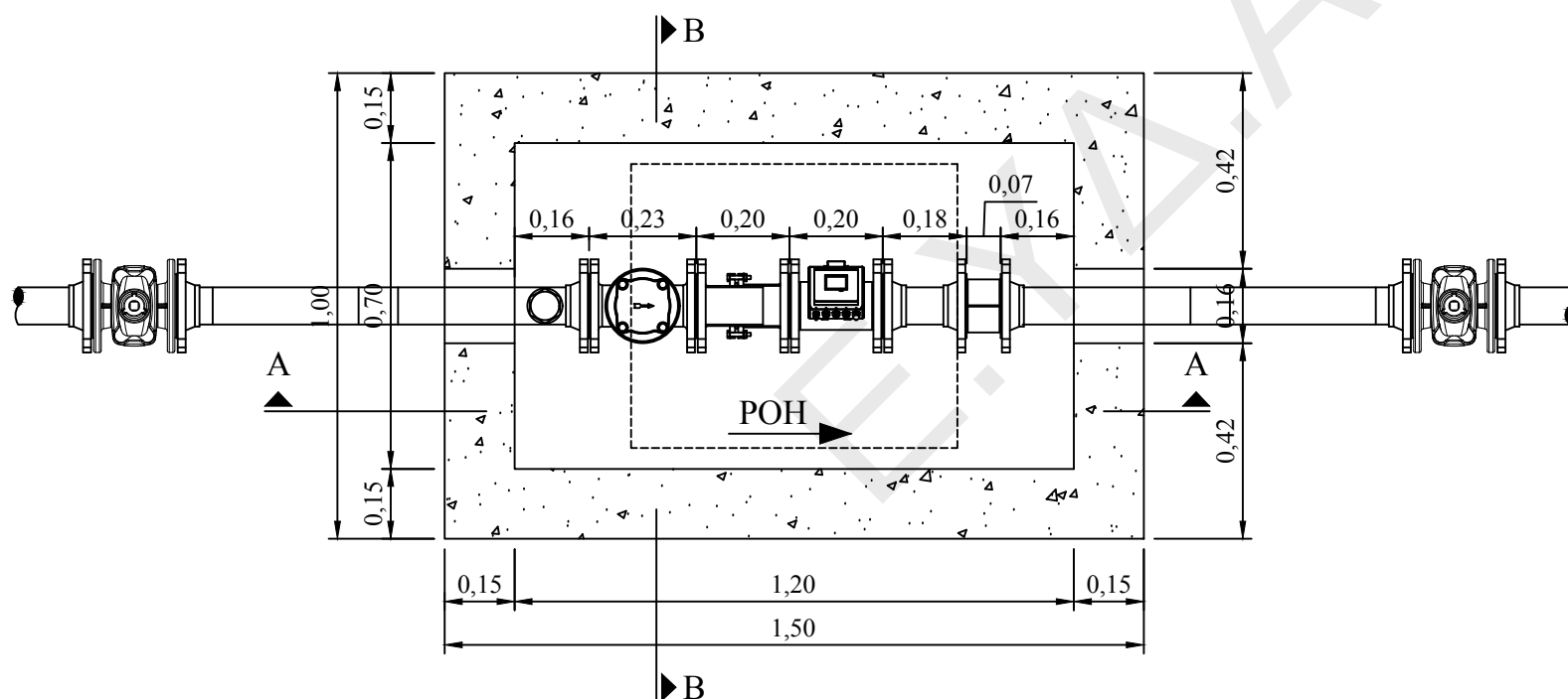
ΚΑΤΟΨΗ
