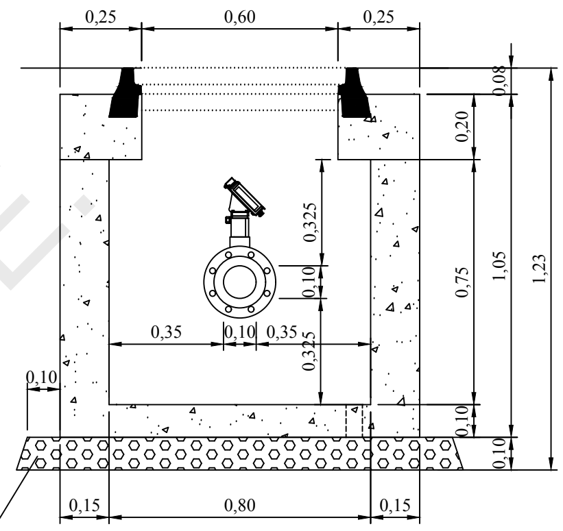
ΤΟΜΗ Β-Β
