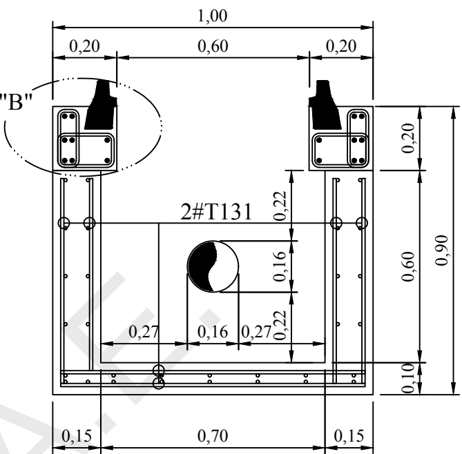
ΤΟΜΗ Β-Β
