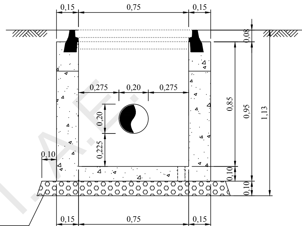
ΤΟΜΗ Β-Β
