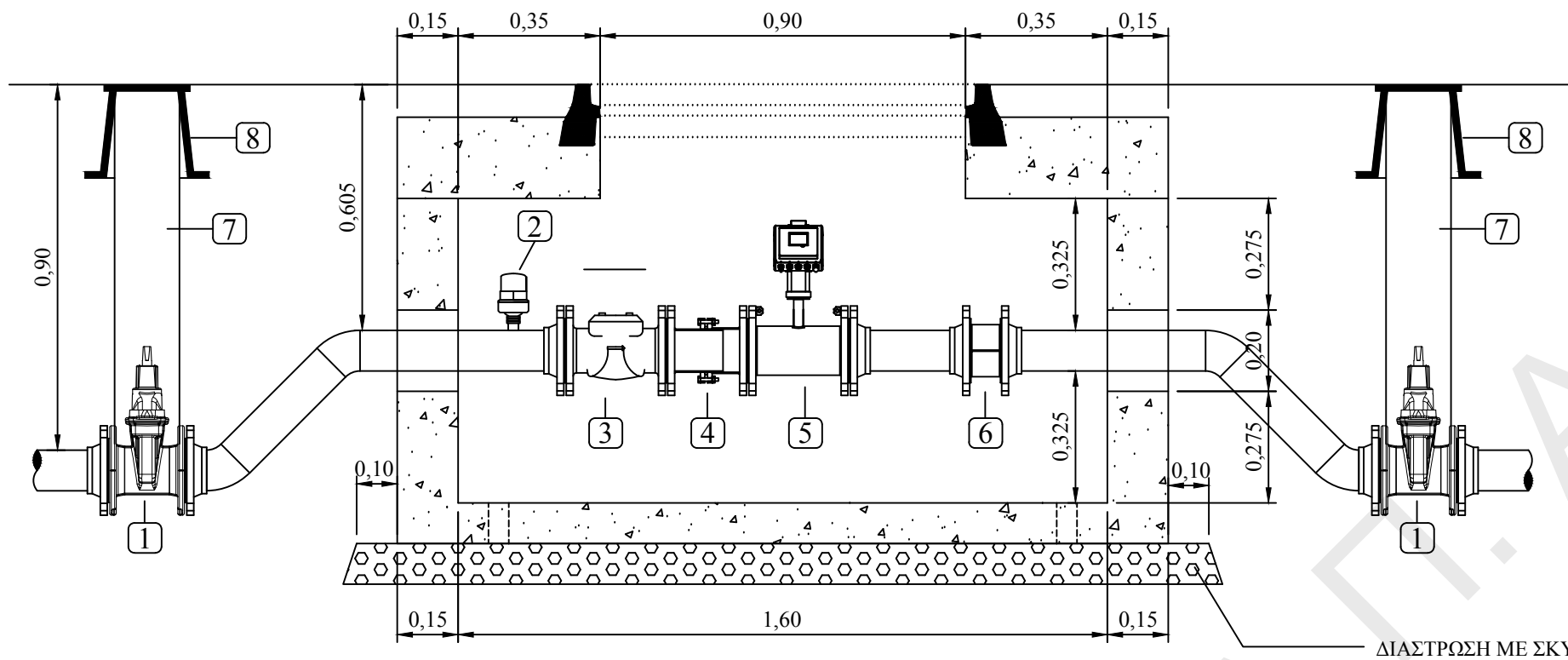
ΤΟΜΗ Α-Α
